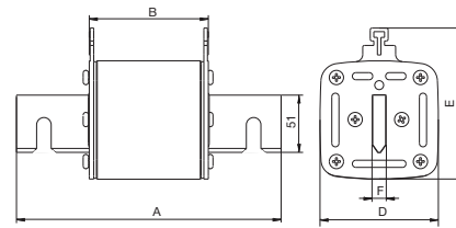
ППН-41
