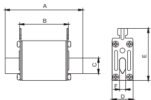
ППН-33 габарит 0
