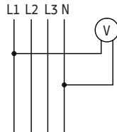
Вольтметр при измерении фазного напряжения
