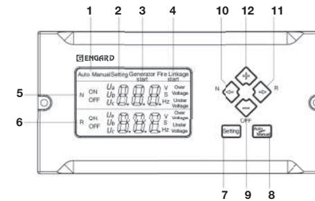
Панель универсального контроллера с ЖК-дисплеем
