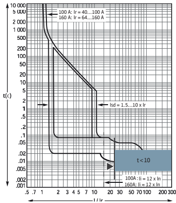
Электронные расцепители ER2, 40-160 A
