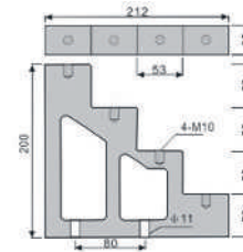
ИС4-50
