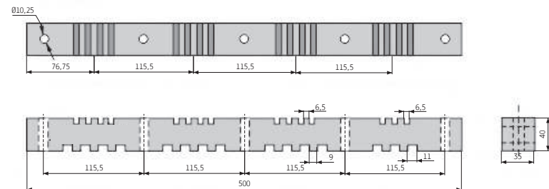
ИШП 4P 500 мм
