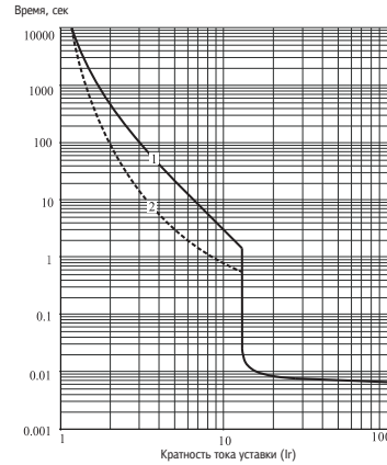
АПД-08 25-80 А
