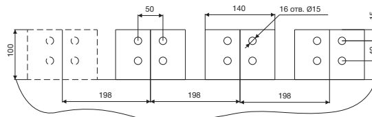
Силовые выводы E5K-3L
