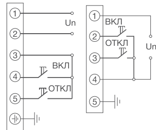
ED2KR-3/6
