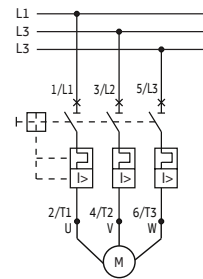
Подключение трехфазного двигателя
