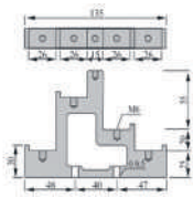
ИС4-25
