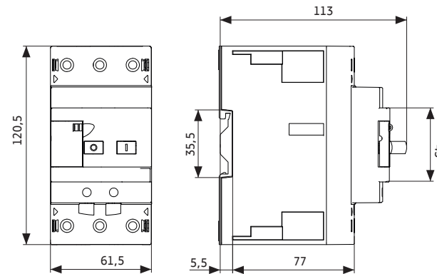
АПД-08 25-80 А
