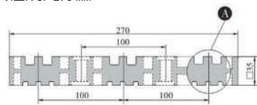
ИШП 3P 270 мм
