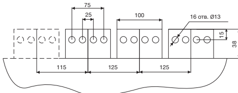
Силовые выводы E5K-2L
