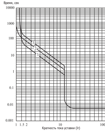
АПД-03 0,16-32 А
