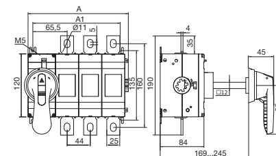
ВНК-3734
