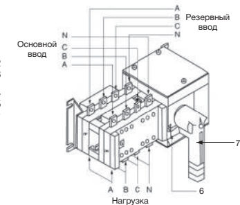
800-3200 A
