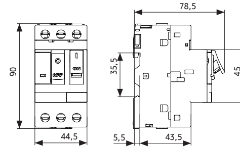
АПД-03 0,16-32 А
