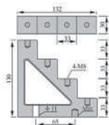
ИС4-30
