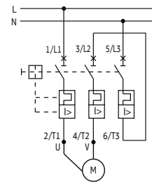
Подключение однофазного двигателя
