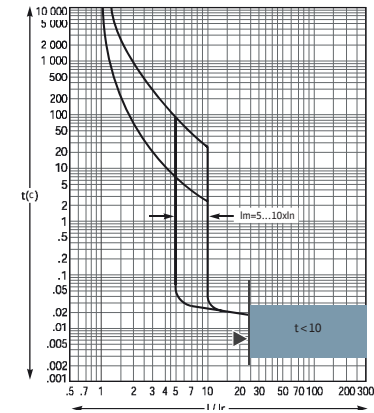
Термомагнитные расцепители TMR, 200-250 A
