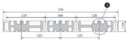
ИШП 2P 180 мм
