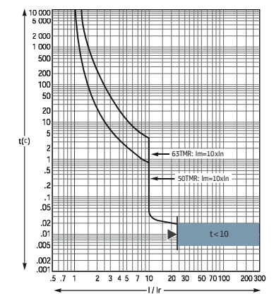
Термомагнитные расцепители TMR, 50-63 A
