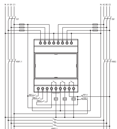
ETS-3ZC
