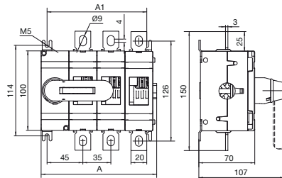
ВНК-3533
