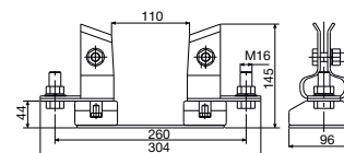
ДП-41
