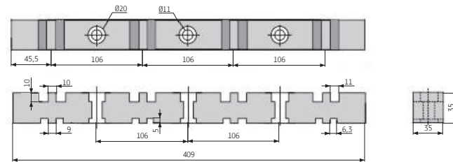
ИШП 4P 409 мм
