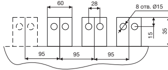
Силовые выводы E5K-1F
