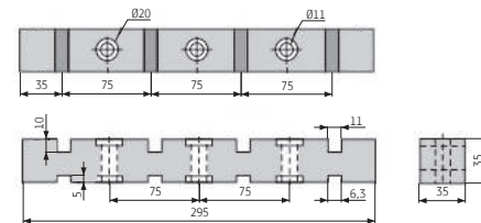
ИШП 4P 295 мм
