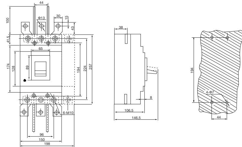
BA88-39
