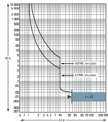
Термомагнитные расцепители TMR, 32-40 A
