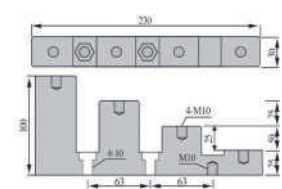
ИСв4-40
