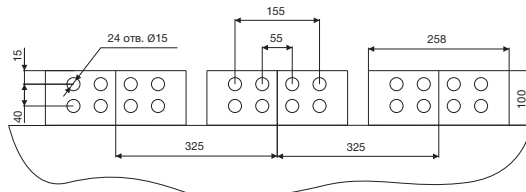
Силовые выводы E5K-4V 6300 A
