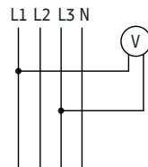
Вольтметр при измерении линейного напряжения
