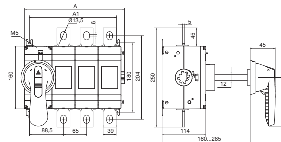
ВНК-3934
