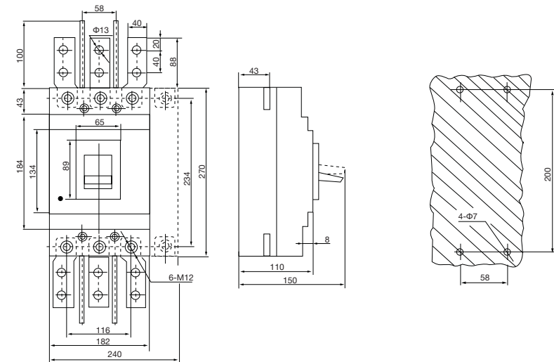
BA88-39
