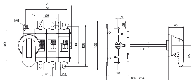
ВНК-3534
