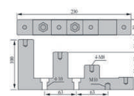
ИСв4-30
