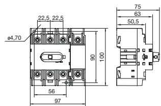
ВНК-3534
