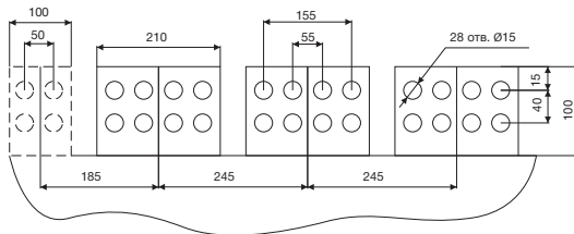
Силовые выводы E5K-4V 5000 A
