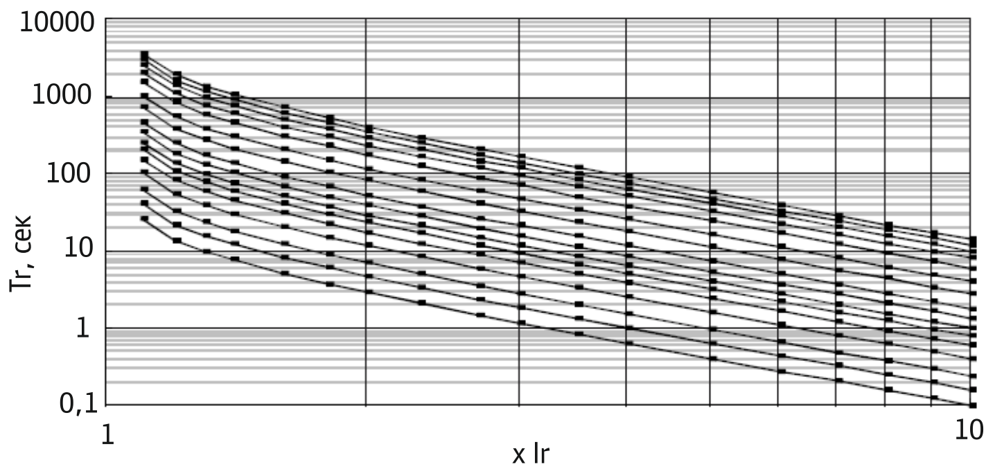
Защита от перегрузки. Кривая срабатывания 4
