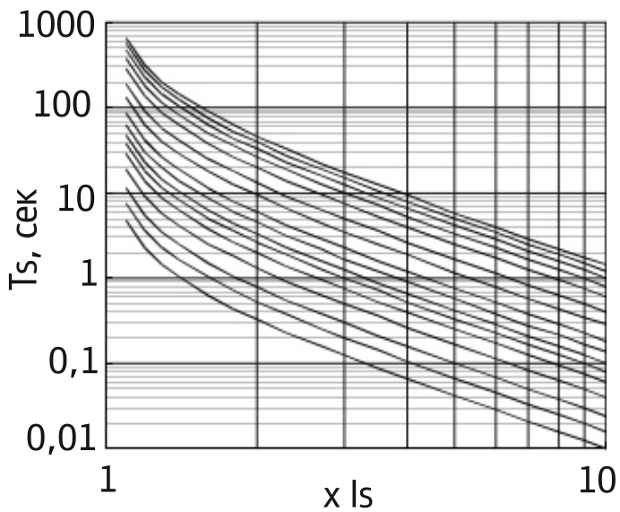
Кривая срабатывания 5
