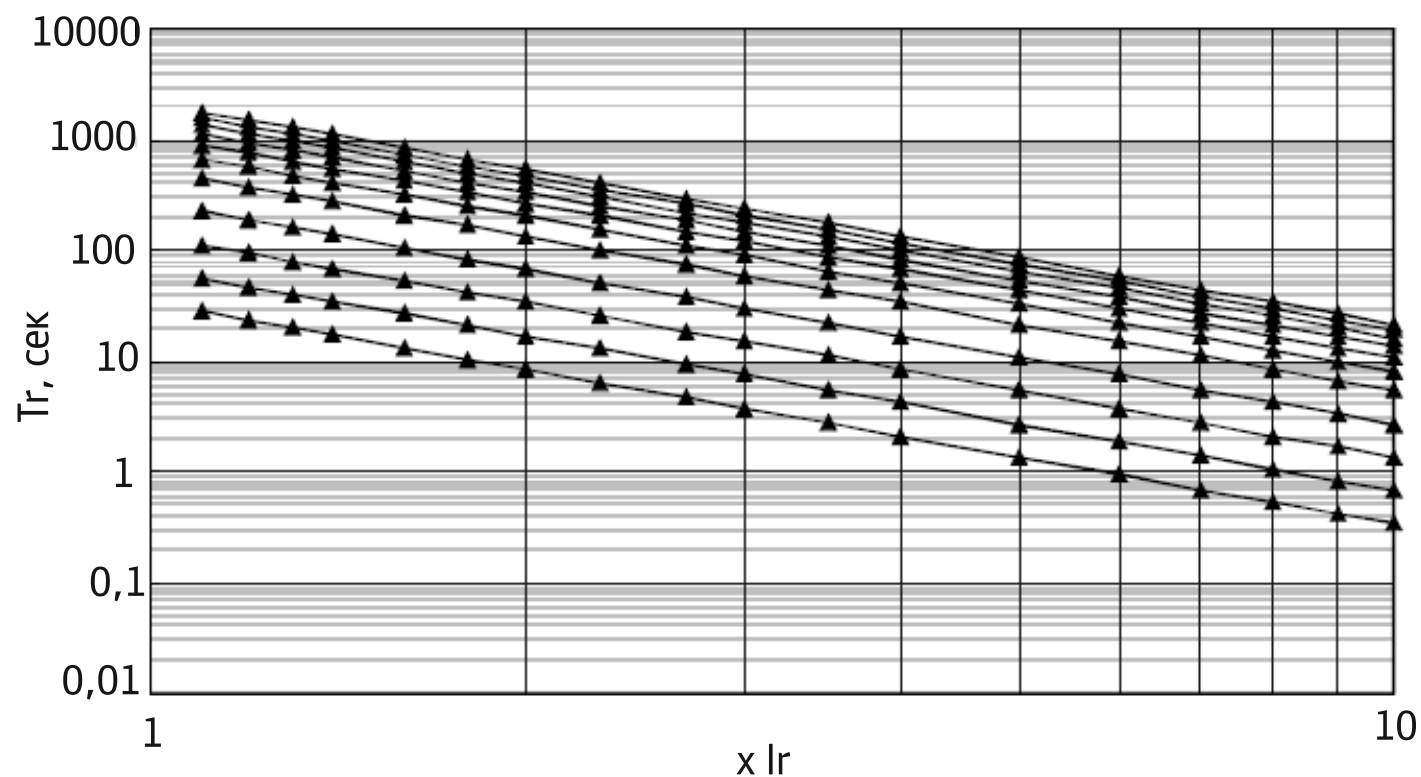
Защита от перегрузки. Кривая срабатывания 6
