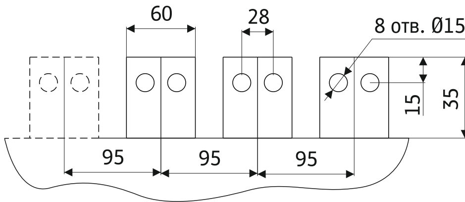
Силовые выводы E5K-1F
