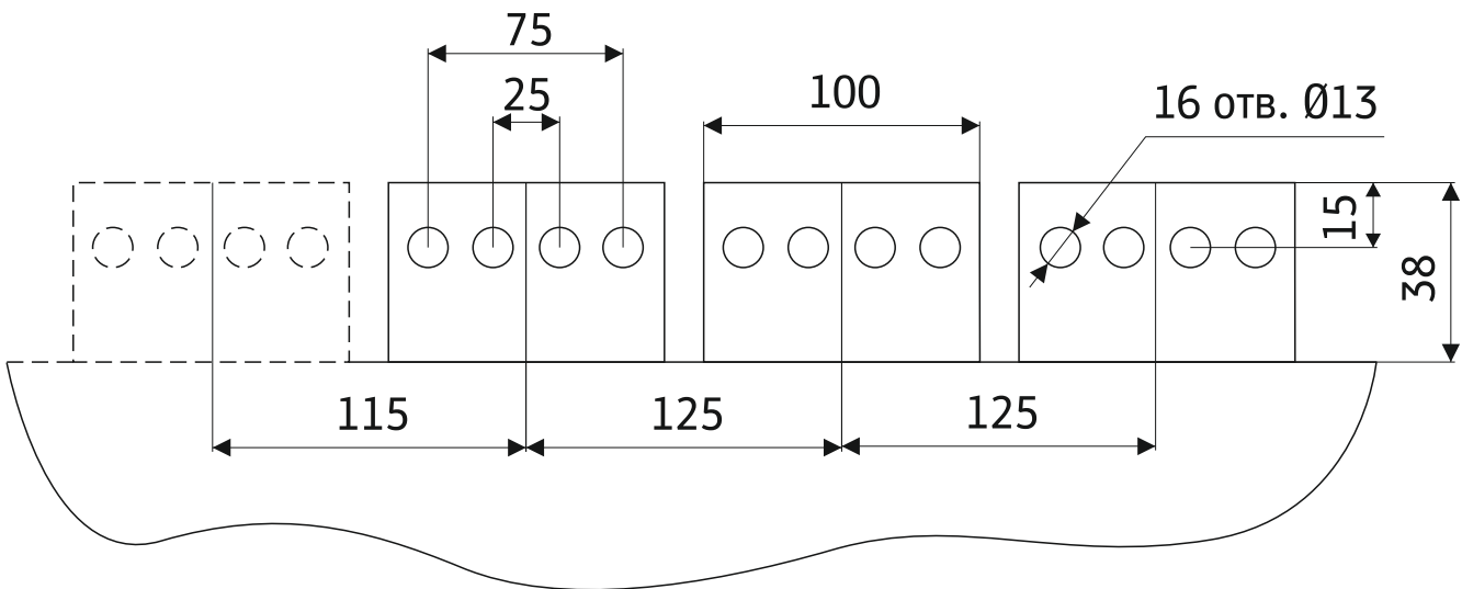
Силовые выводы E5K-2L
