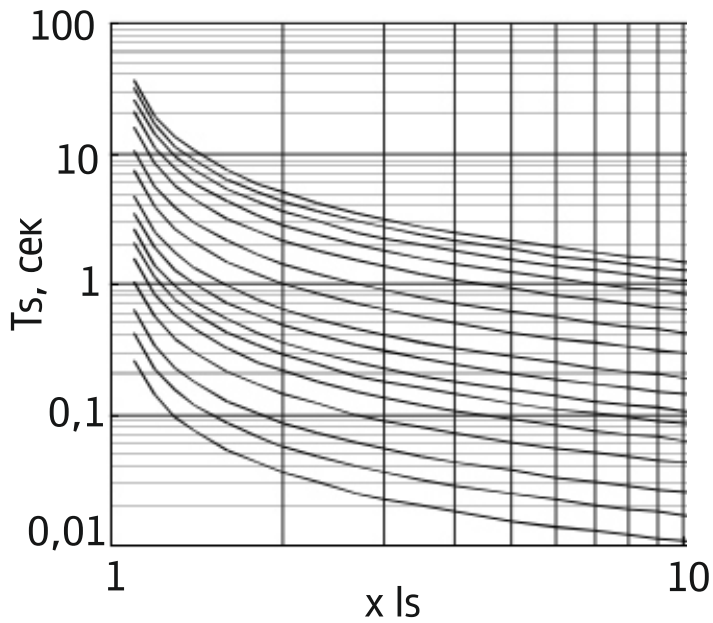
Кривая срабатывания 3
