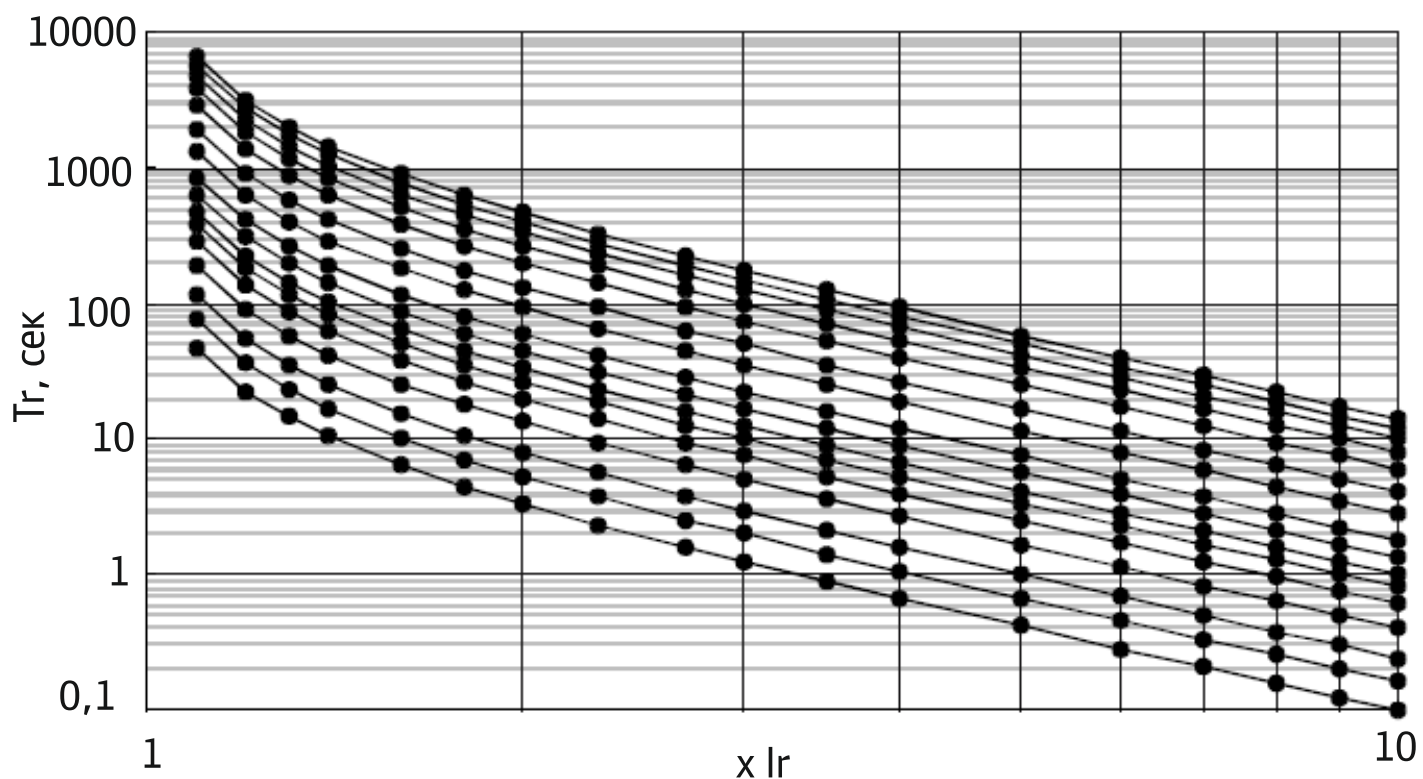
Защита от перегрузки. Кривая срабатывания 3
