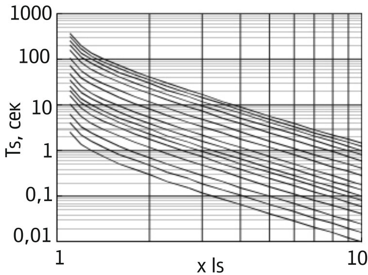
Кривая срабатывания 6
