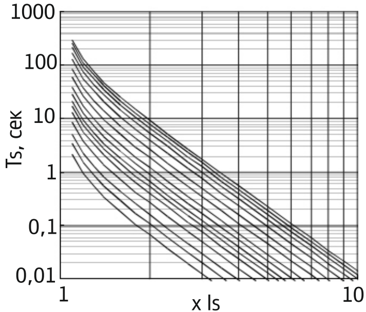
Кривая срабатывания 5
