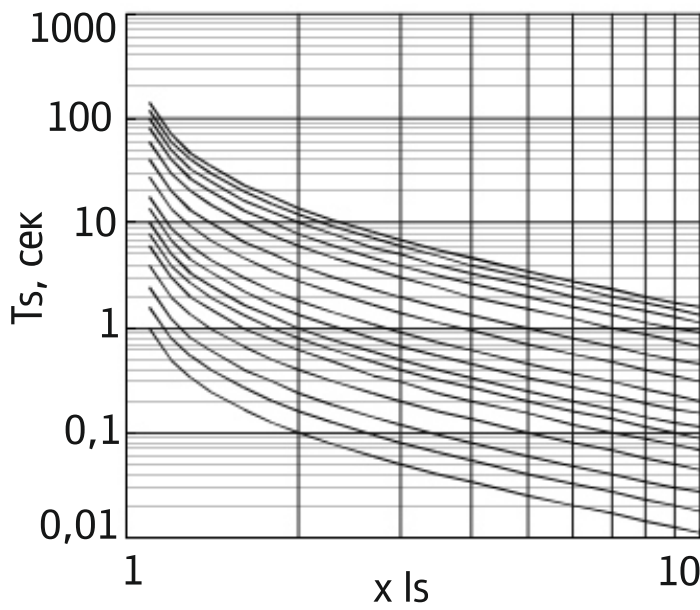
Кривая срабатывания 4
