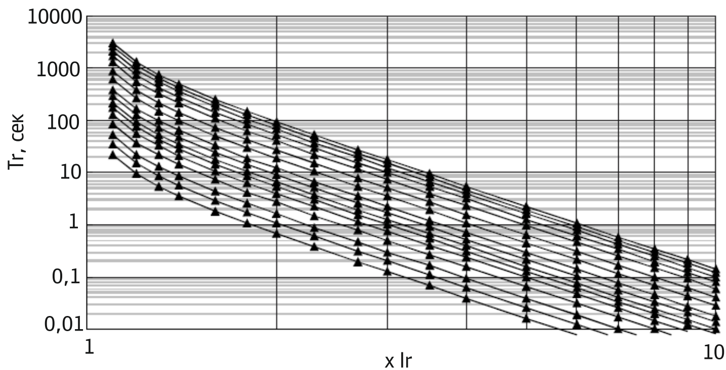
Защита от перегрузки. Кривая срабатывания 5
