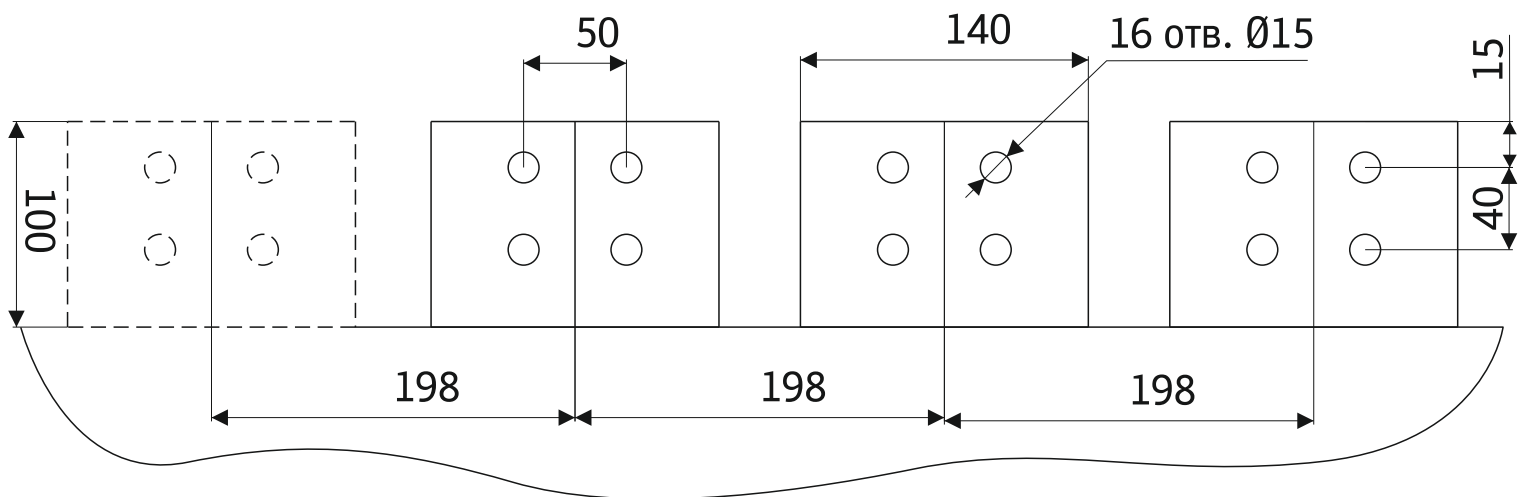
Силовые выводы E5K-3L 4000 A
