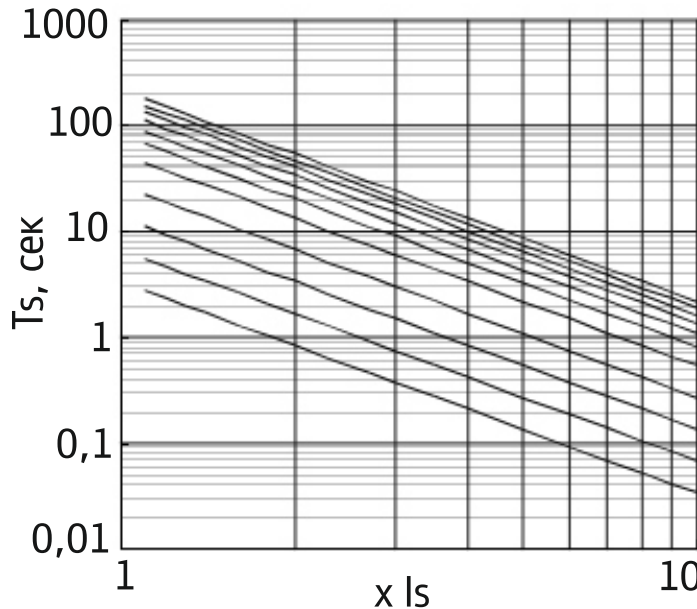
Кривая срабатывания 6
